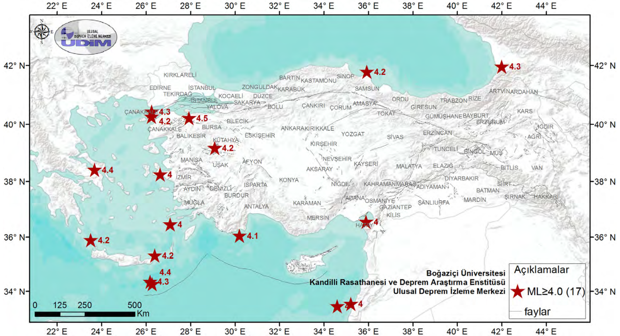
2014 Temmuz ayı Türkiye ve yakın çevresi M \geq 4.0 olan depremlerin dağılımı
