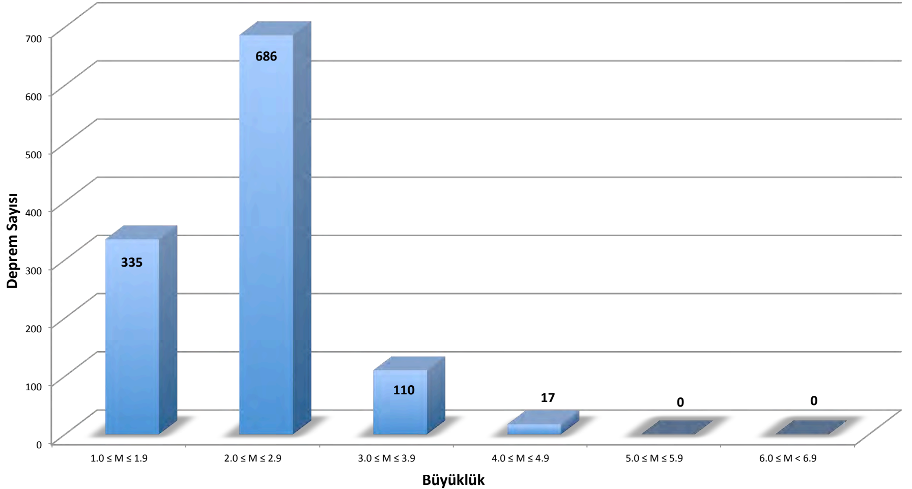
Temmuz 2014 Deprem Sayısı - Büyüklük Dağılım Grafiği
