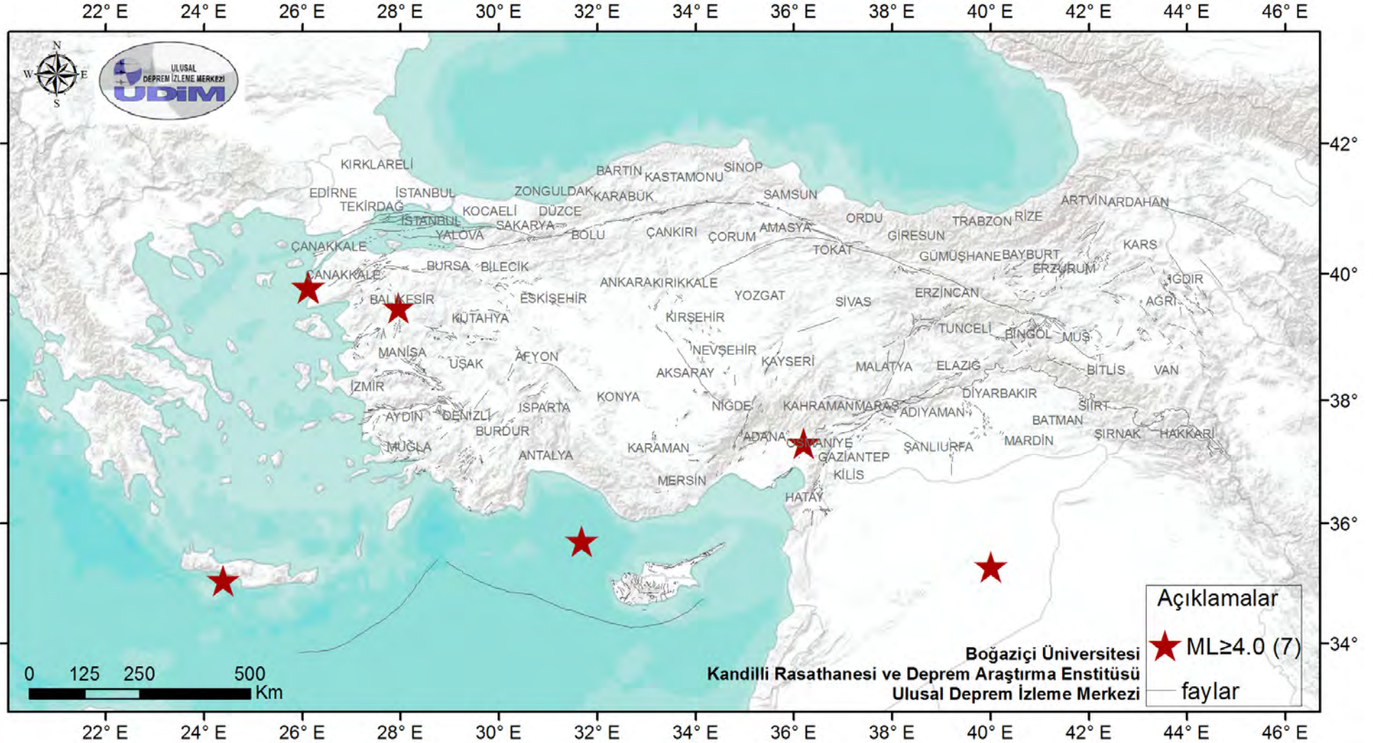
2014 Ocak ayı Türkiye ve yakın çevresi M \geq 4.0 olan depremlerin dağılımı
