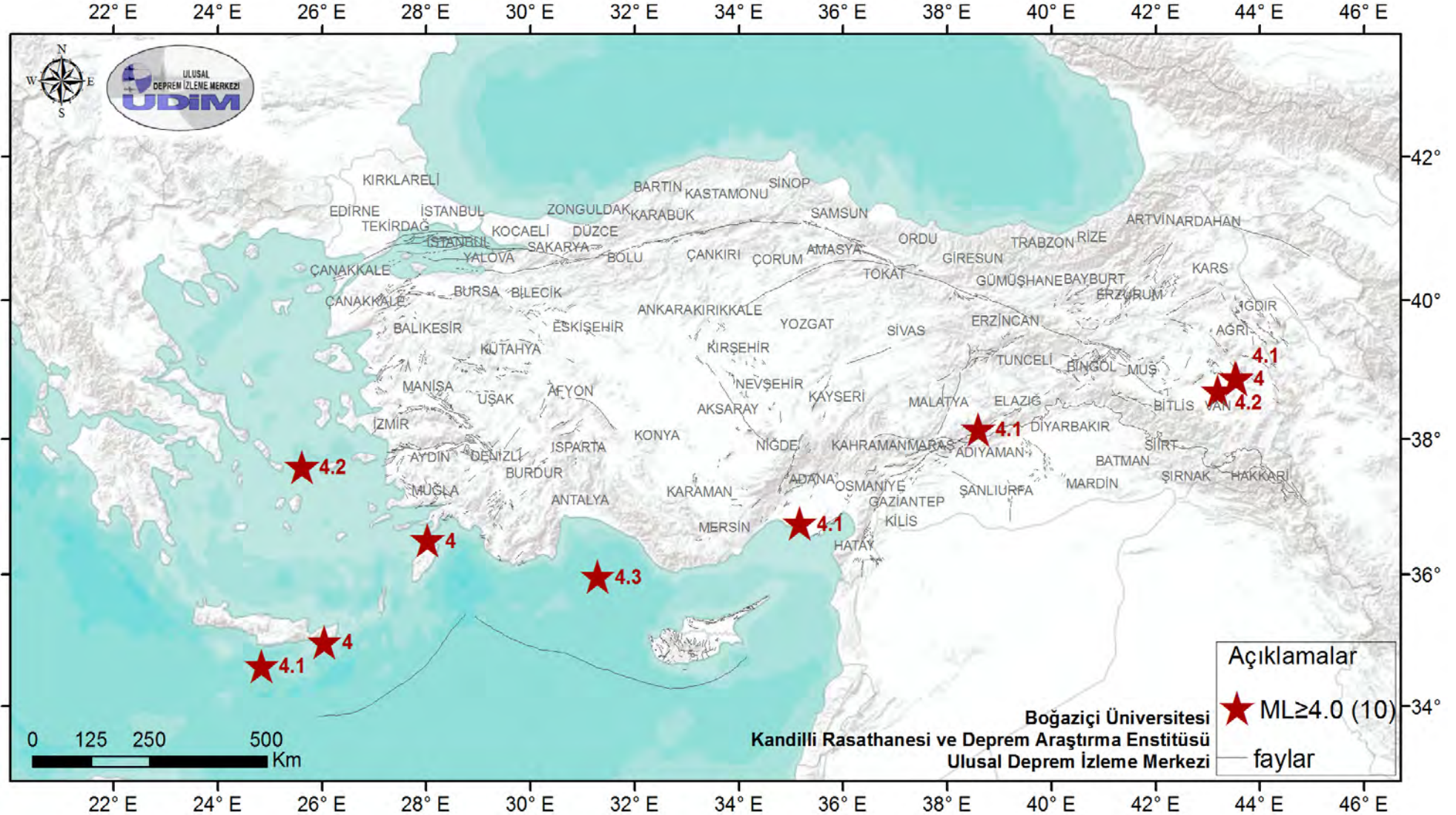
2014 Mart ayı Türkiye ve yakın çevresi M \geq 4.0 olan depremlerin dağılımı
