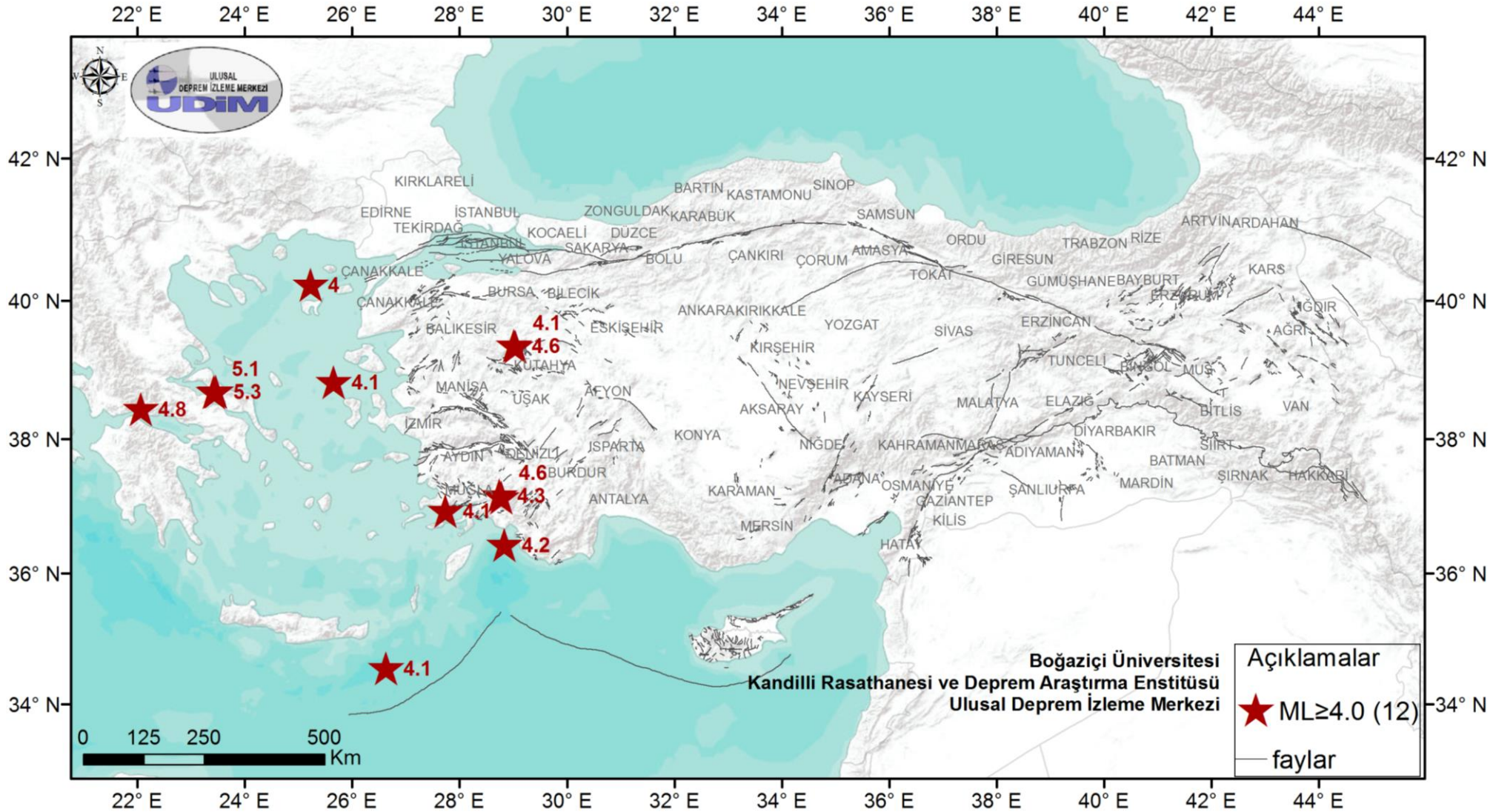
2014 Kasım ayı Türkiye ve yakın çevresi M \geq 4.0 olan depremlerin dağılımı
