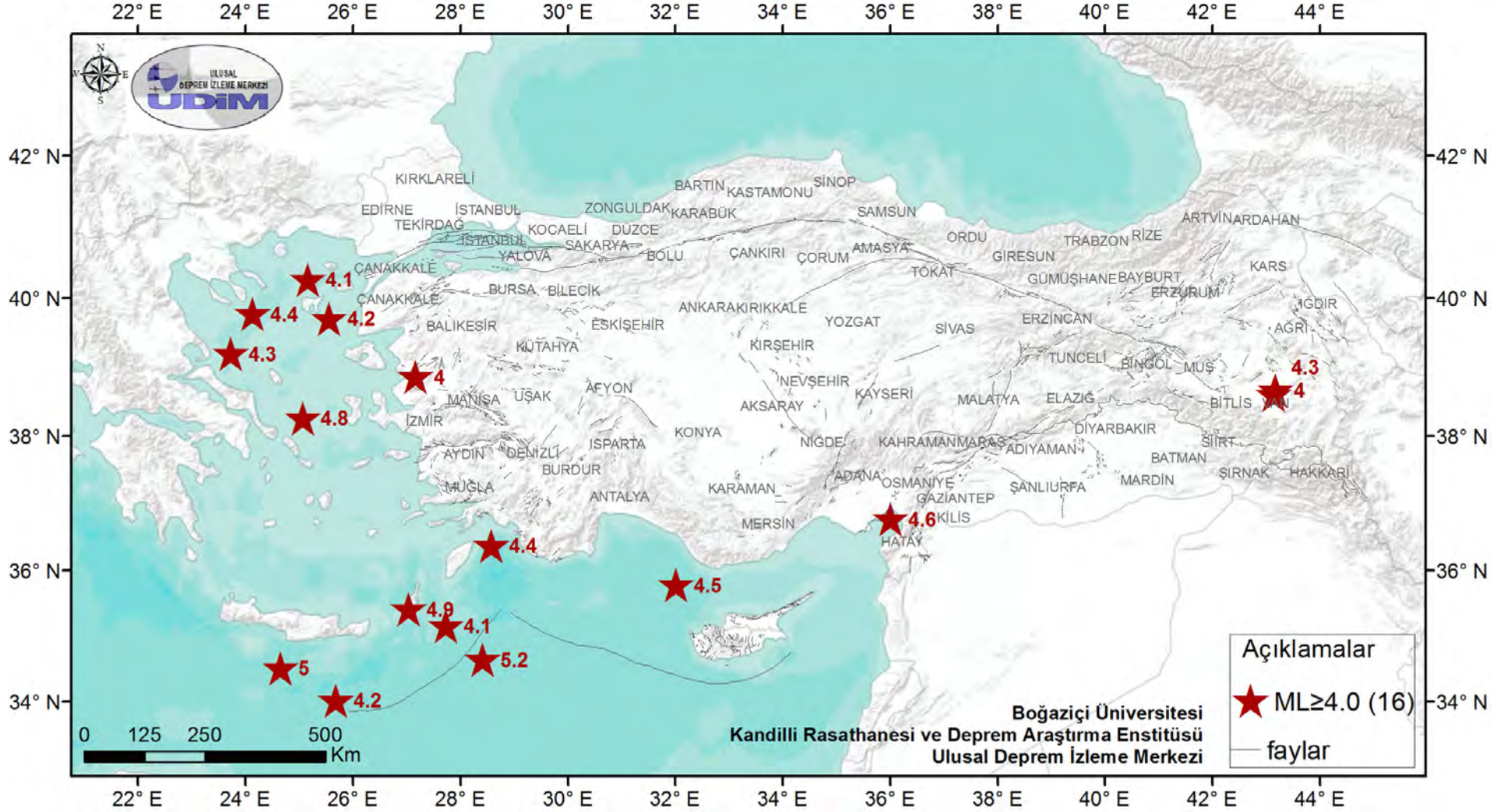
2014 Haziran ayı Türkiye ve yakın çevresi M \geq 4.0 olan depremlerin dağılımı
