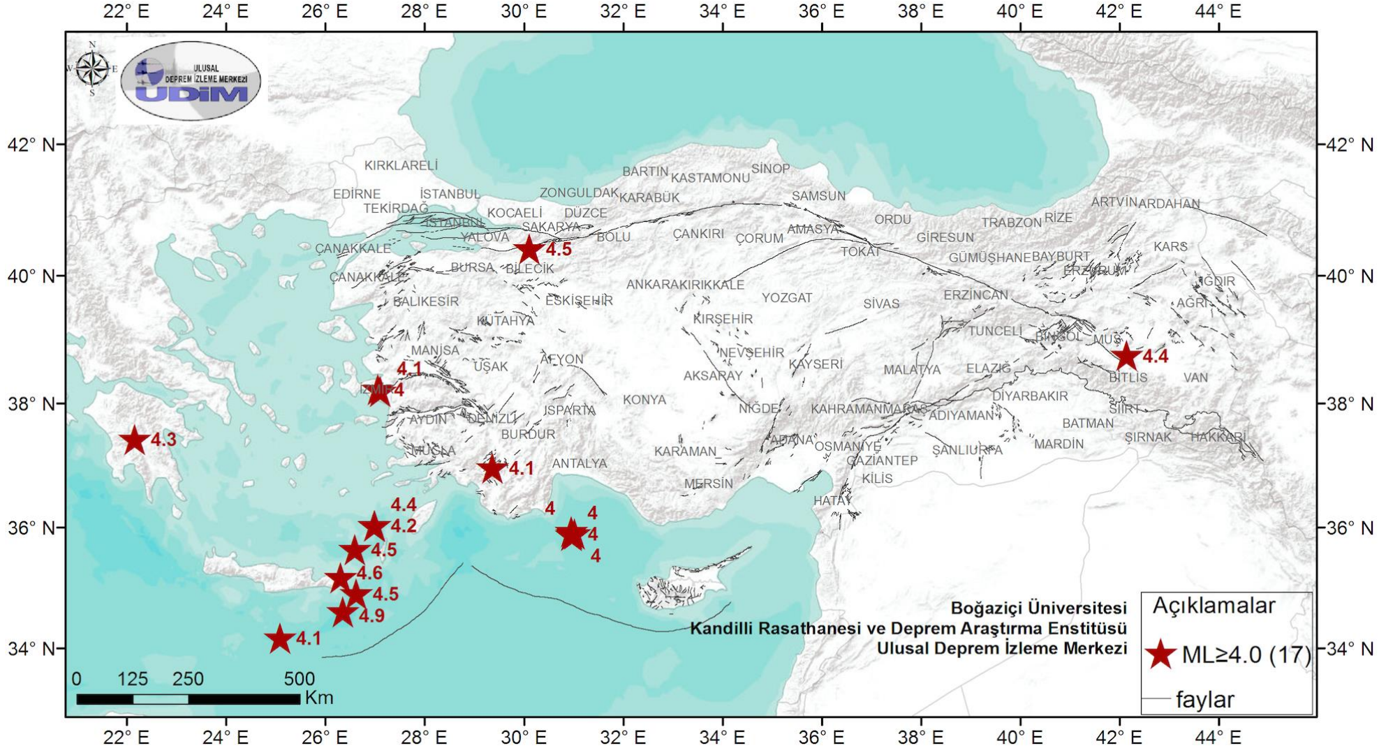
2014 Ekim ayı Türkiye ve yakın çevresi M \geq 4.0 olan depremlerin dağılımı
