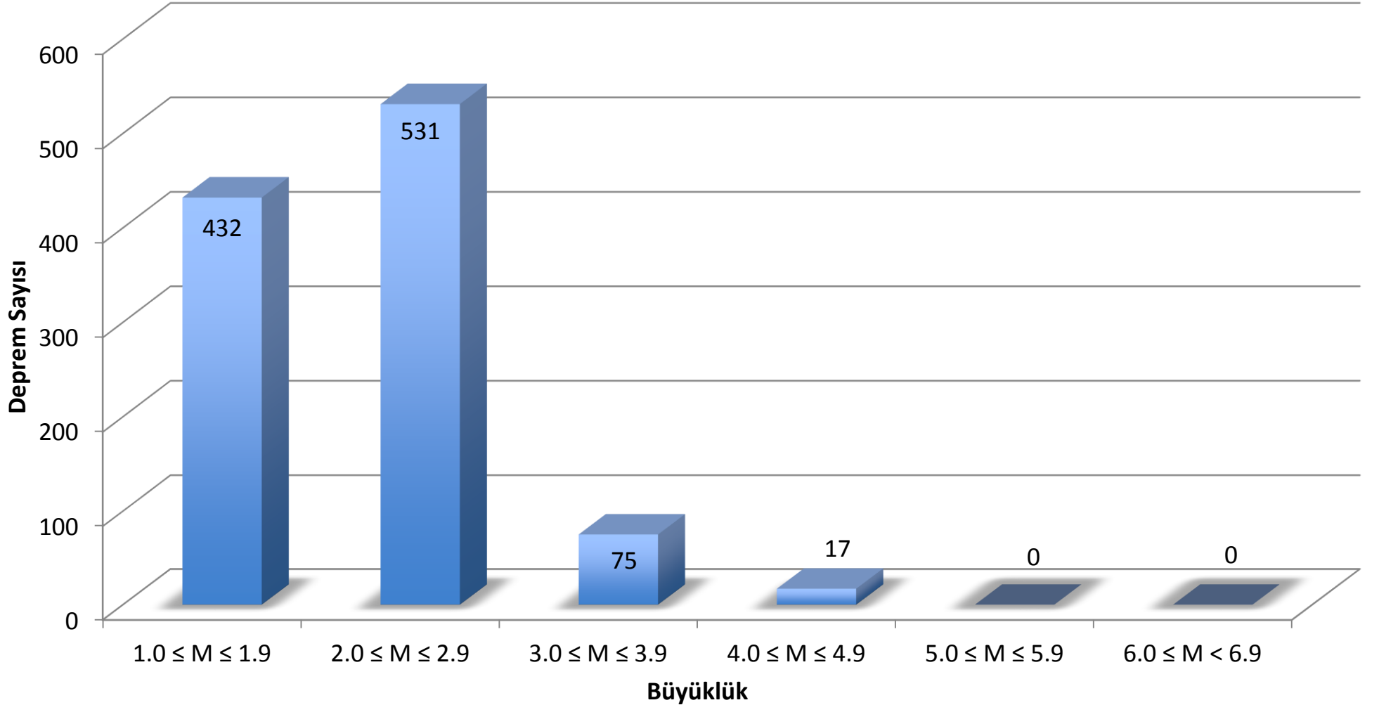
Ekim 2014 Deprem Sayısı - Büyüklük Dağılım Grafiği
