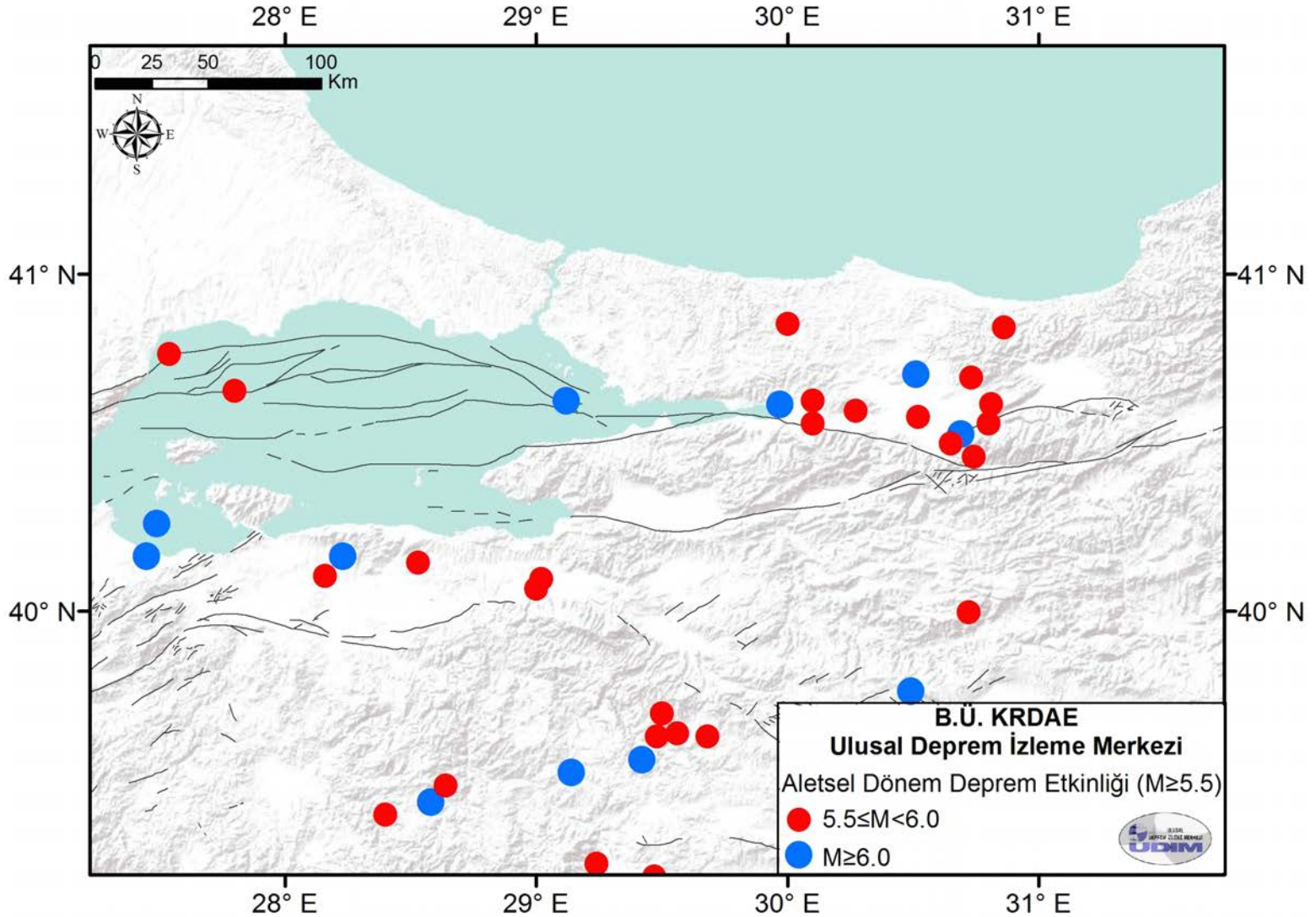
Bölgenin Aletsel Dönem (1900 – 2014) Depremleri
