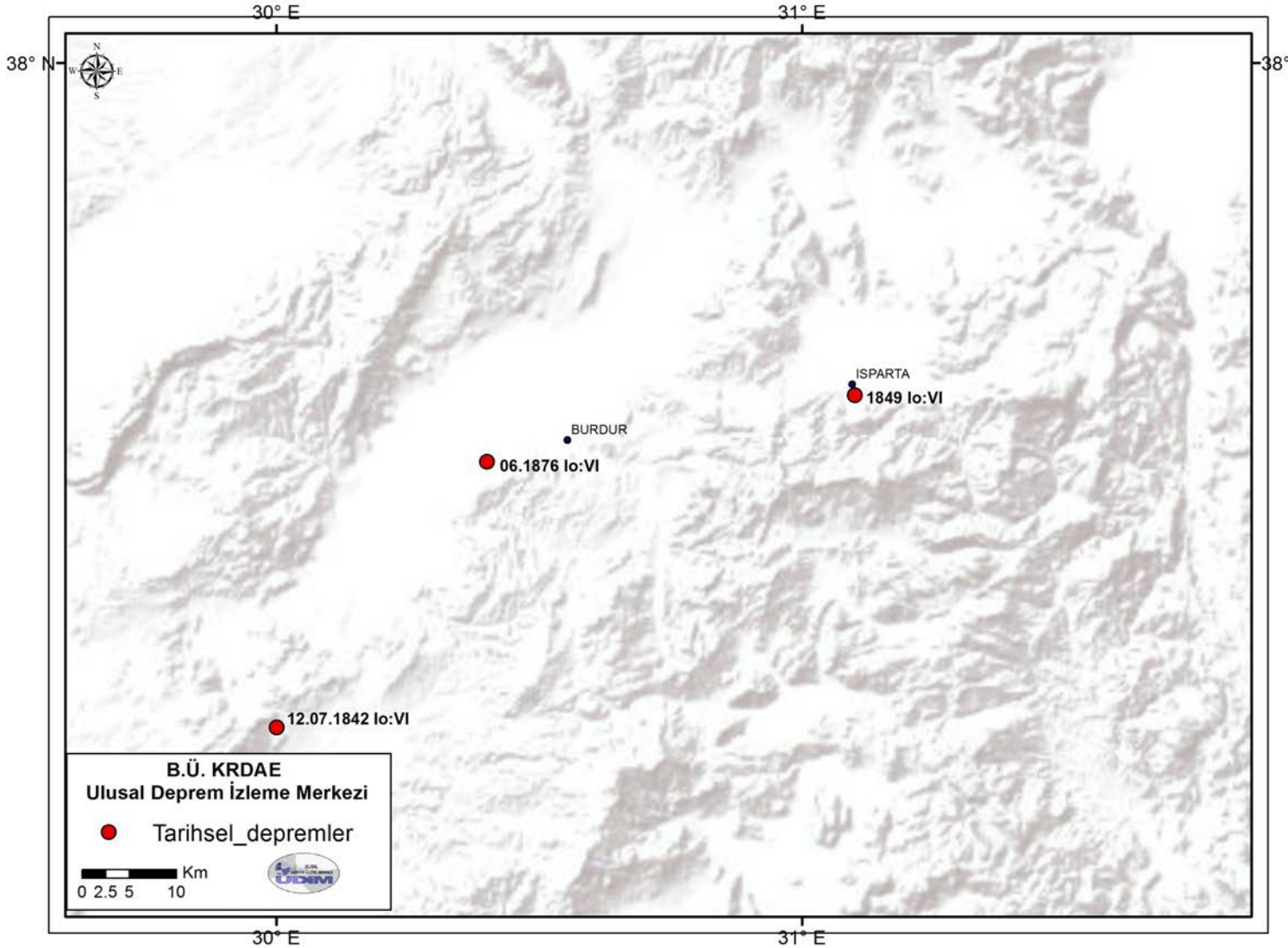
Bölgenin Tarihsel Dönem (1900 Yılı Öncesi) Depremleri
