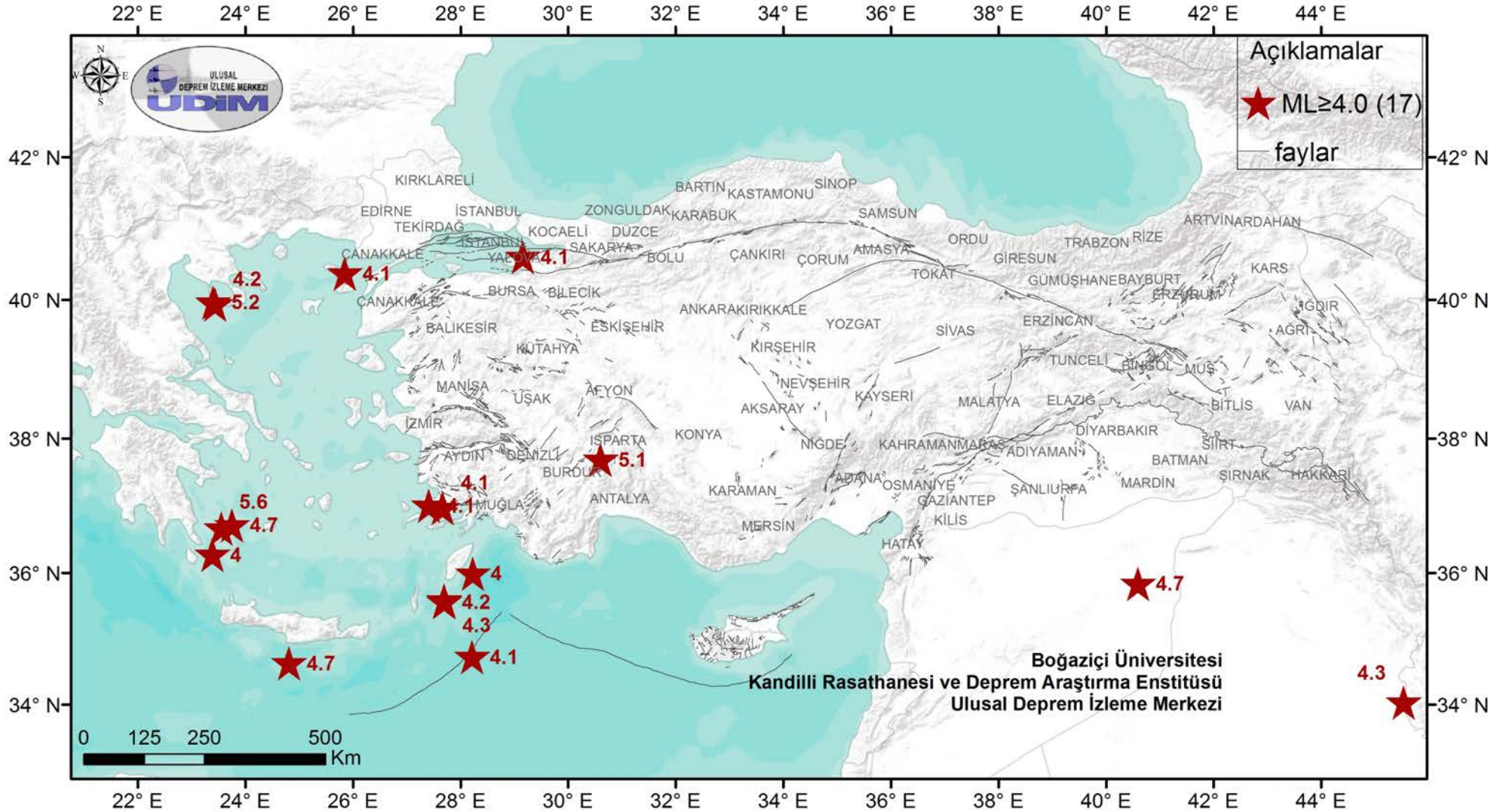
2014 Ağustos ayı Türkiye ve yakın çevresi M \geq 4.0 olan depremlerin dağılımı
