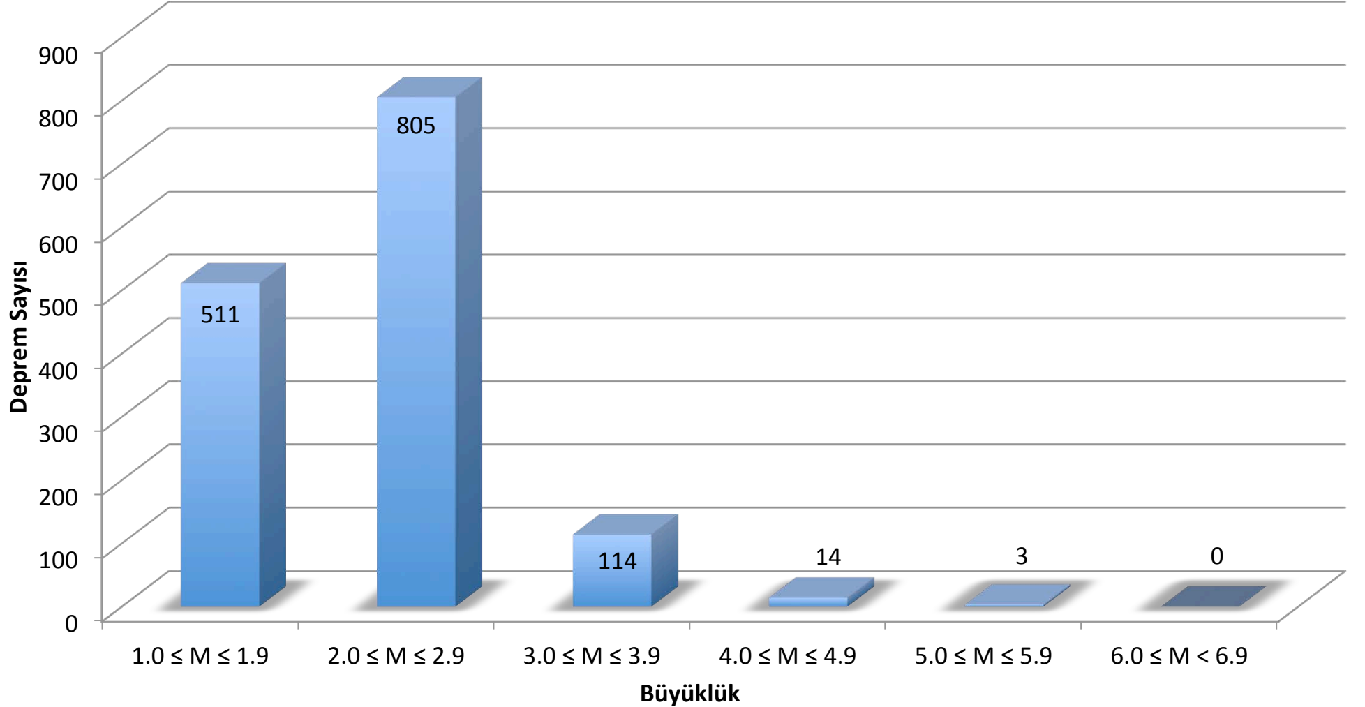
Ağustos 2014 Deprem Sayısı - Büyüklük Dağılım Grafiği
