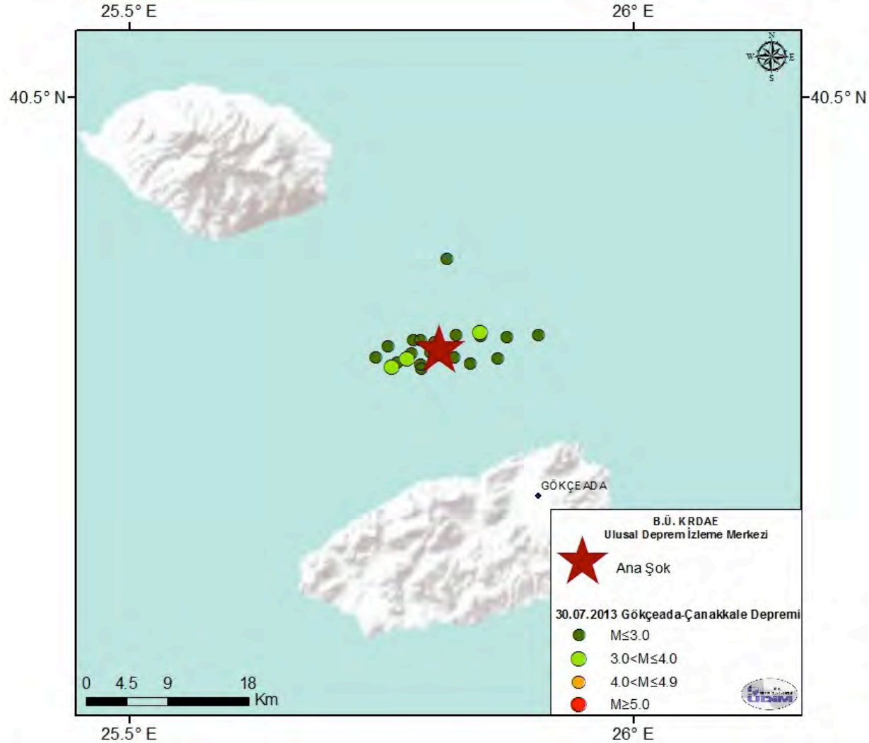
Gökçeada (Çanakkale) Deprem Etkinliği (30-31 Temmuz 2013)
