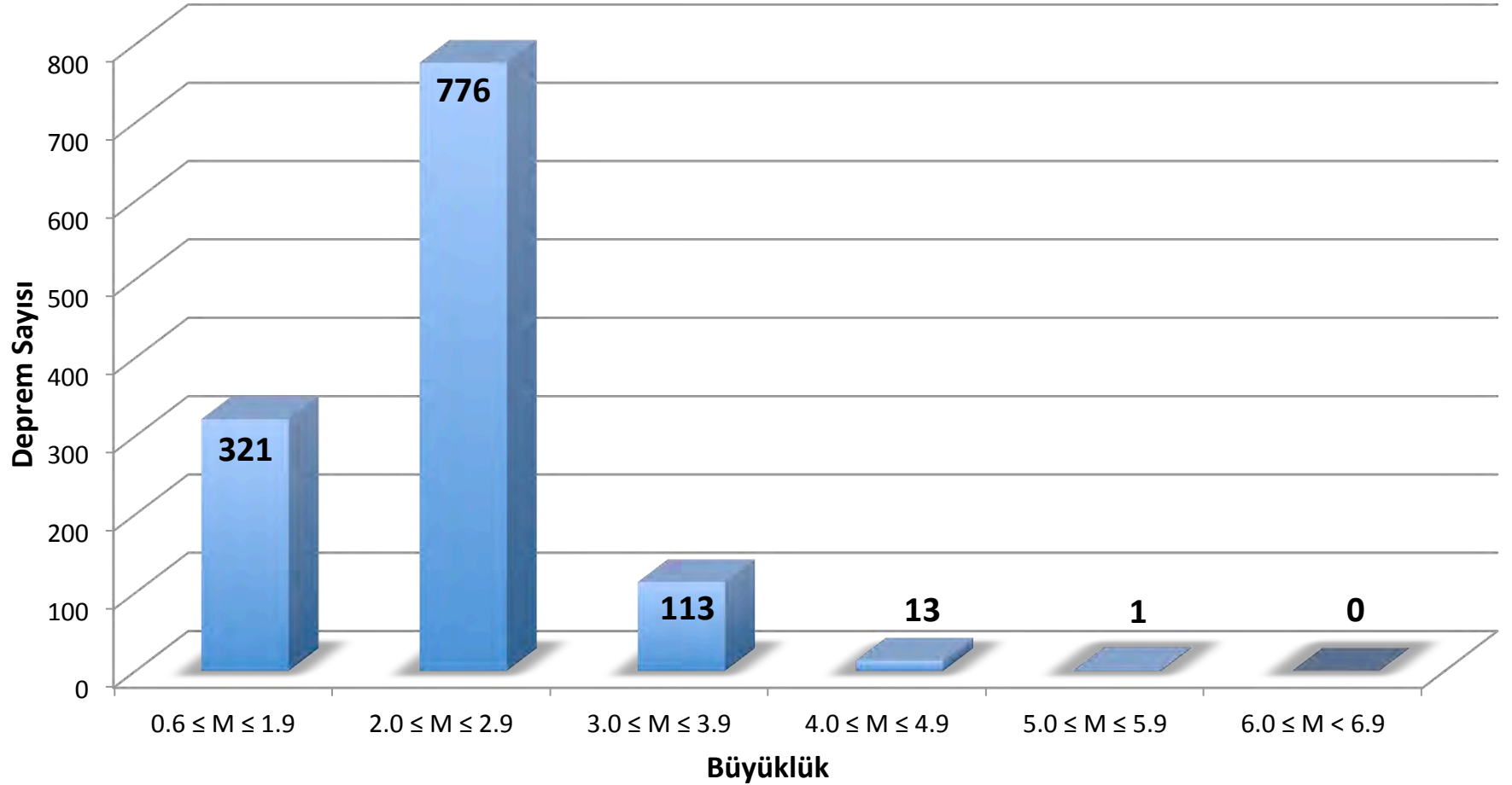
Temmuz 2013 Deprem Sayısı - Büyüklük Dağılım Grafiği
