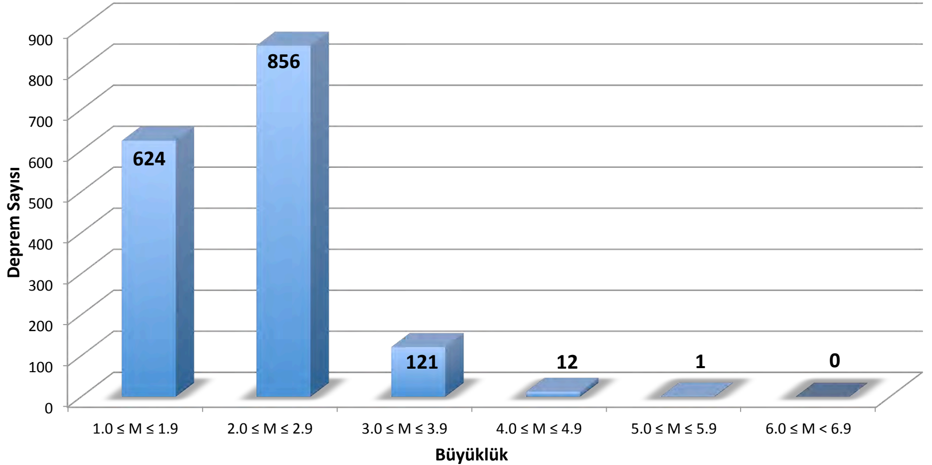
Nisan 2013 Deprem Sayısı - Büyüklük Dağılım Grafiği
