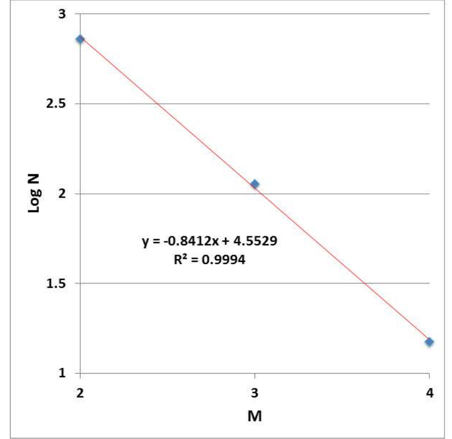
HAZİRAN 2016 TÜRKİYE VE YAKIN ÇEVRESİNİN GUTENBERG-RİCHTER MAGNİTÜD-DEPREM SAYISI GRAFİĞİ
