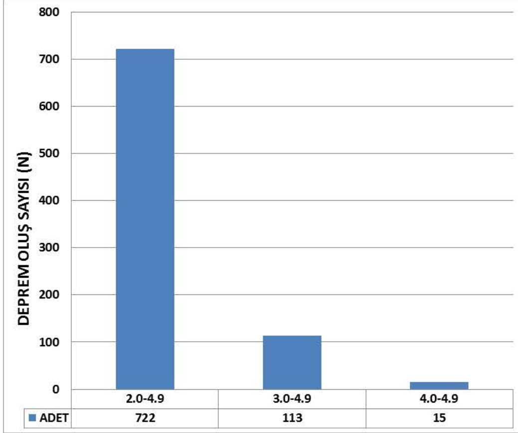
HAZİRAN 2016 TÜRKİYE VE YAKIN ÇEVRESİNİN GUTENBERG-RİCHTER MAGNİTÜD-DEPREM SAYISI GRAFİĞİ
