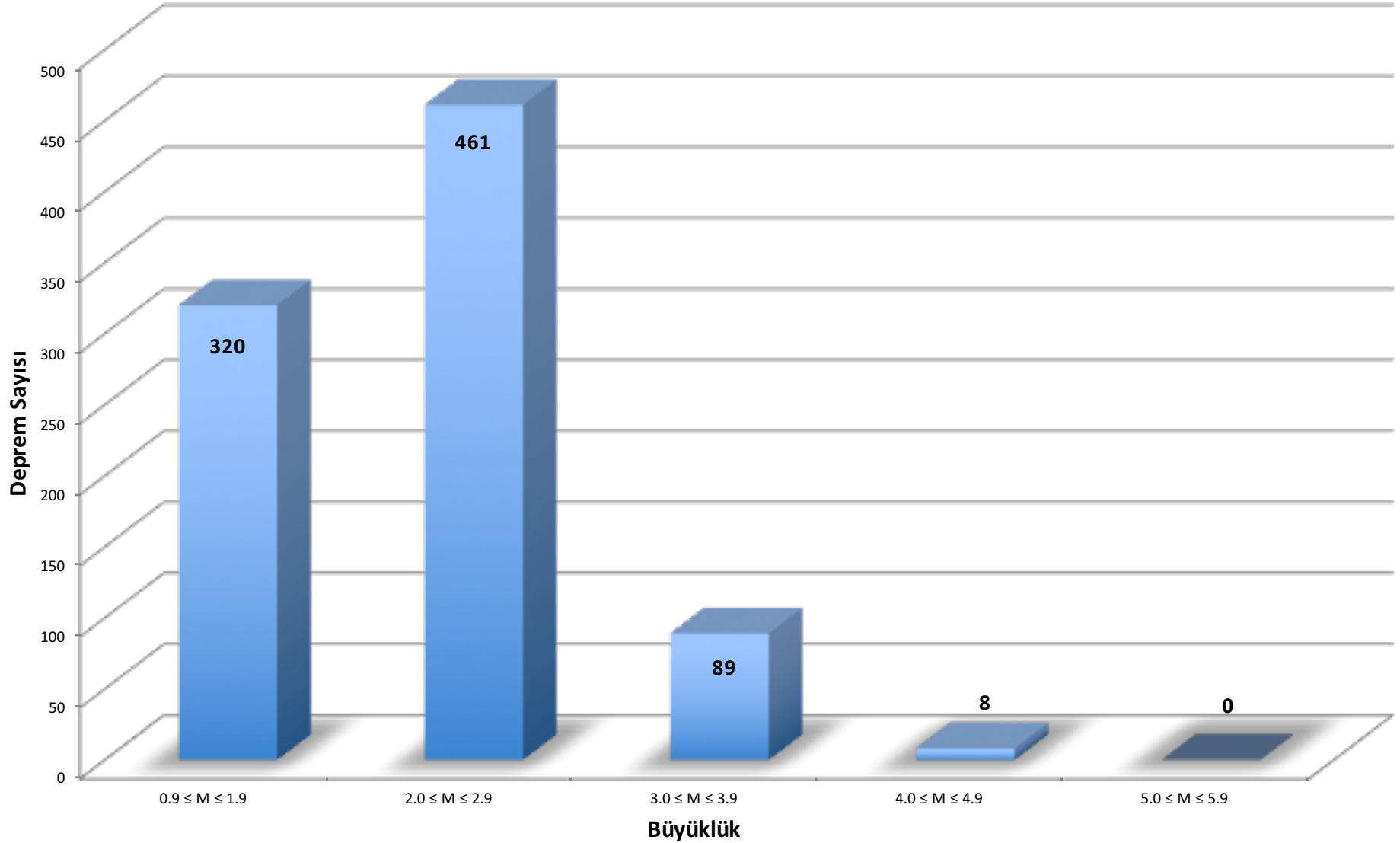
Şubat 2016 Deprem Sayısı - Büyüklük Dağılım Grafiği
