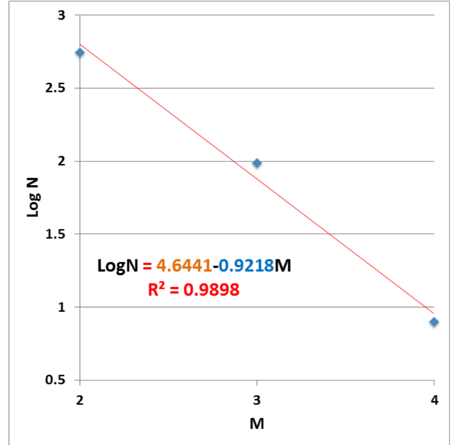
ŞUBAT 2016 TÜRKİYE VE YAKIN ÇEVRESİNİN GUTENBERG-RİCHTER MAGNİTÜD-DEPREM SAYISI GRAFİĞİ
