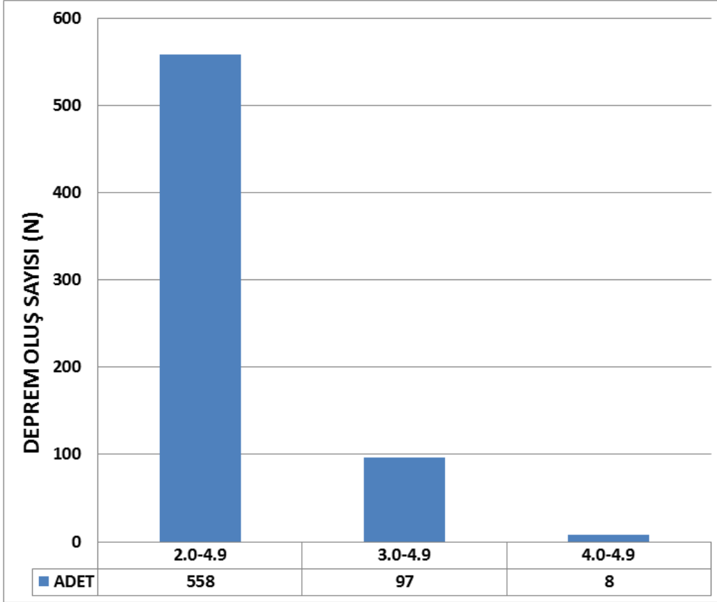
ŞUBAT 2016 TÜRKİYE VE YAKIN ÇEVRESİNİN GUTENBERG-RİCHTER MAGNİTÜD-DEPREM SAYISI GRAFİĞİ
