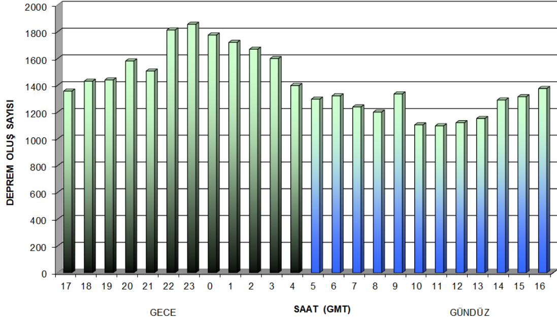
2017 YILINDA DEPREMLERİN SAATLERE GÖRE DAĞILIMI ( 0.2 ≤ M ≤ 7.2 )
