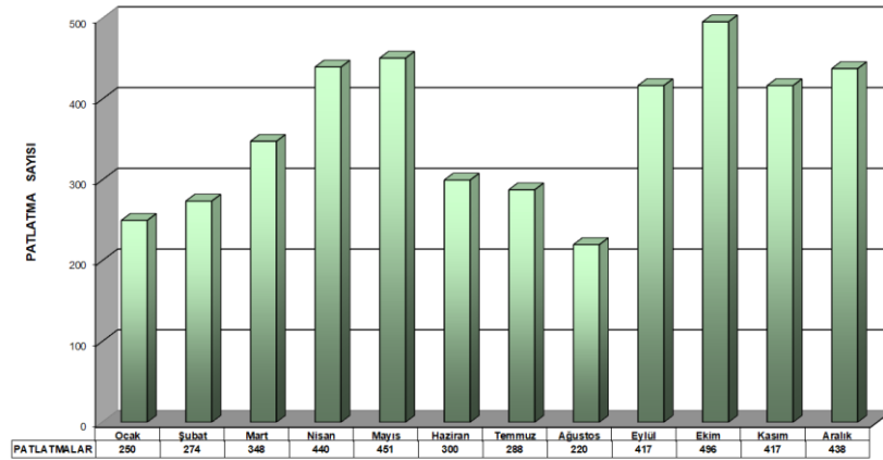
2017 YILINDA İNSAN KAYNAKLI PATLATMALARIN AYLARA GÖRE DAĞILIMI TOPLAM : 4339 Adet
