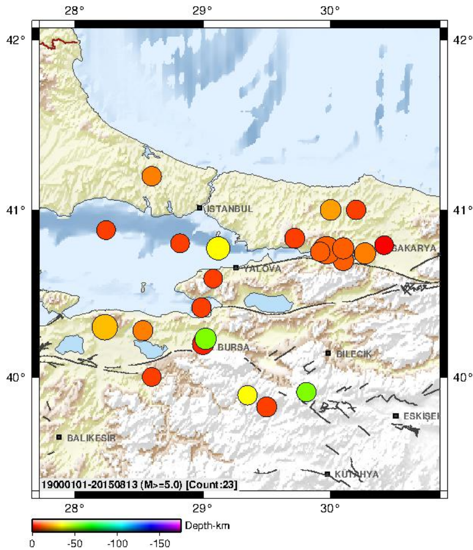
Bölgenin Aletsel Dönem Deprem Etkinliği (M \geq 5.0)
