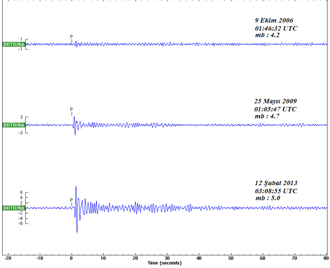
Şekil 9: KKDHC 2006, 2009 ve 2013 nükleer denemelerinin BRTR’da kaydedilen sinyallerinin genlik karşılaştırması
