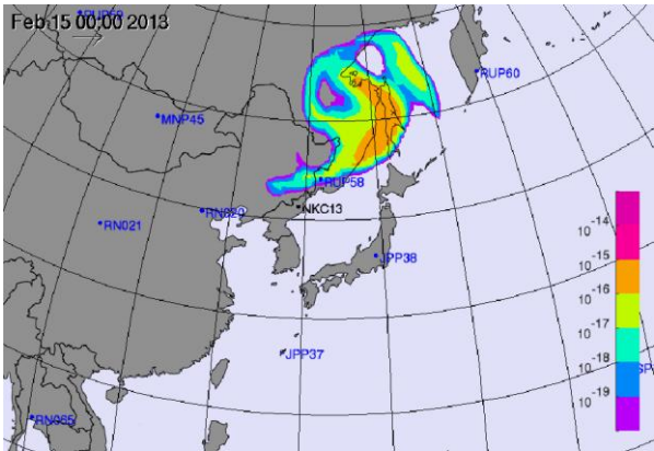
Şekil 8: KKDHC Nükleer Denemesine ait CTBTO tarafından üretilmiş olan Atmosferik Transfer Modelleri (14 Şubat 00:00 UTC – 15 Şubat 12:00 UTC)
